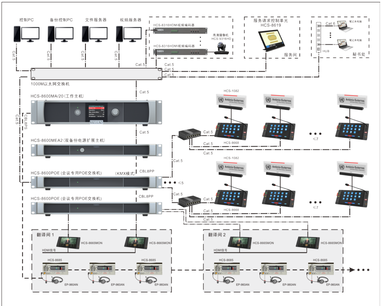
图 1.1.5 HCS-8668/50 系列台式无纸化多媒体会议系统连接图 (PoE 供电)
