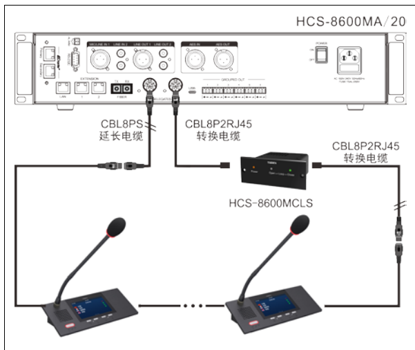
图 2.1.4 会议系统主机与会议单元（8P-DIN）的环形连接
