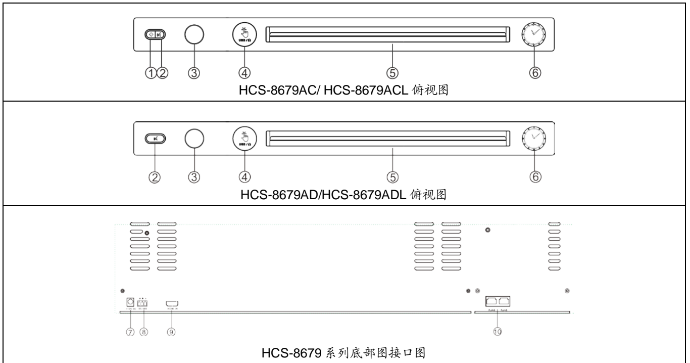
图 3.2.4 HCS-8679 系列无纸化多媒体会议终端
