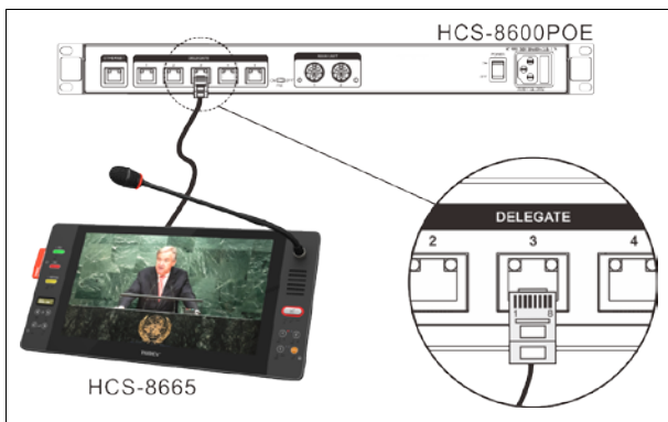
图 3.3.3 HCS-8665 系列简约型多媒体会议终端的连接
