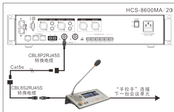
图 4.2.2 HCS-8685 翻译单元与会议控制主机或扩展主机的连接 2
