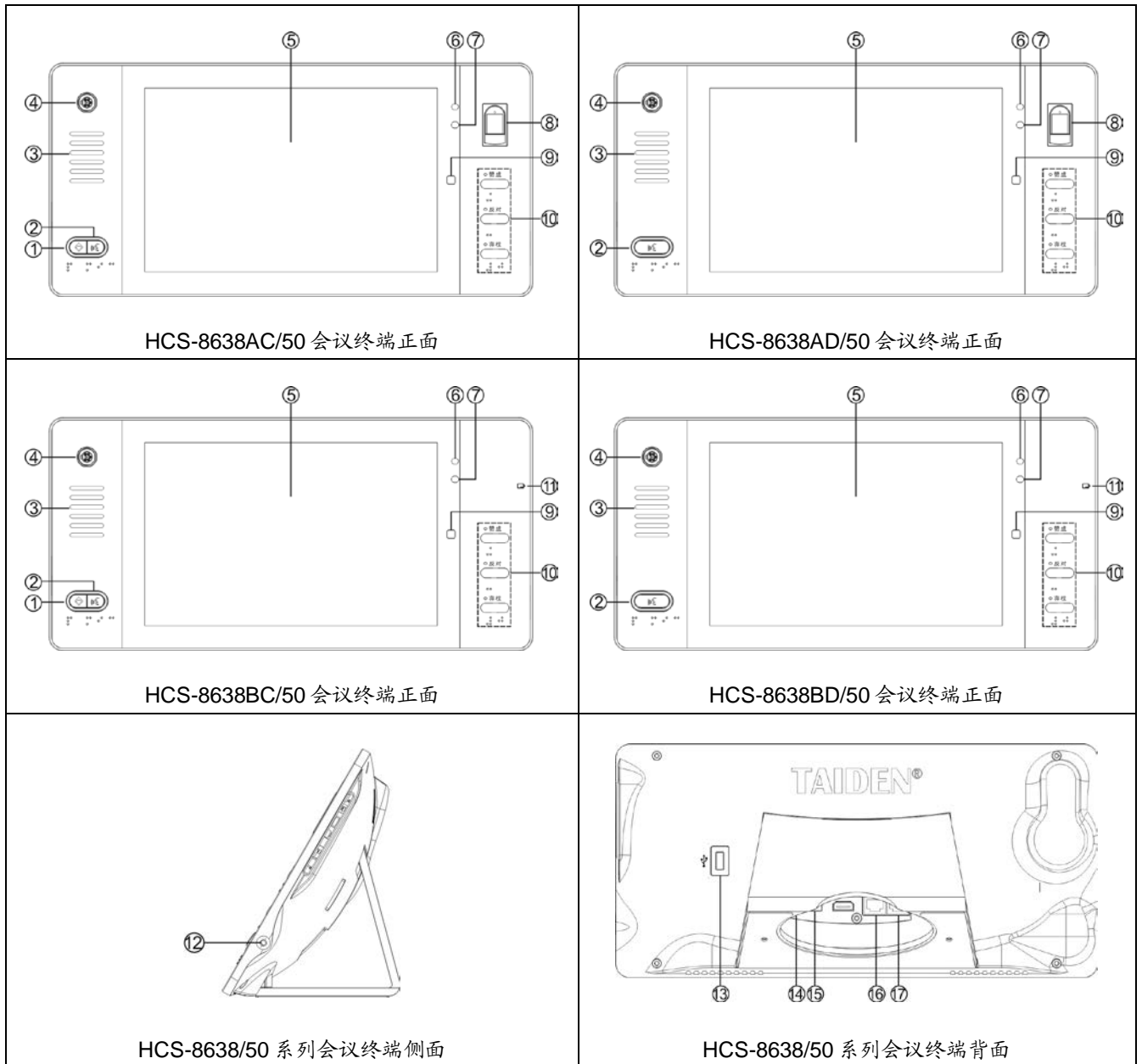
图 3.2.2 HCS-8638/50 系列无纸化多媒体会议终端
