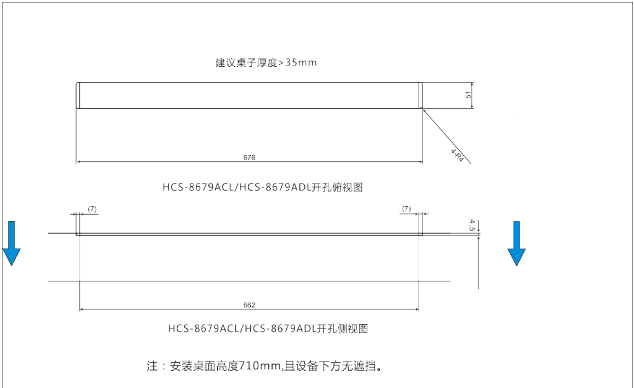
图 3.2.9 HCS-8679L 系列无纸化多媒体会议终端桌面嵌入安装 (单位: mm)
