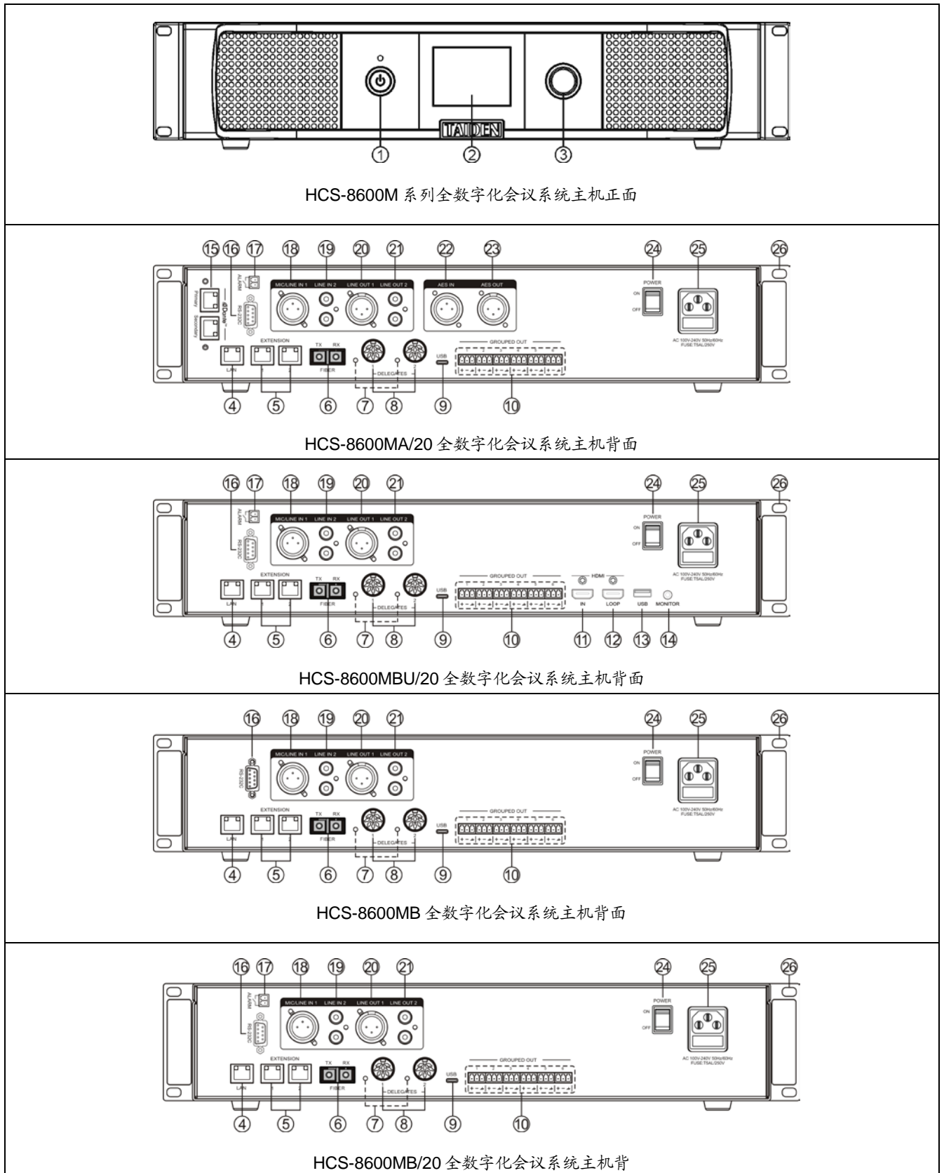
图 2.1.1 HCS-8600M 系列全数字化会议系统主机
