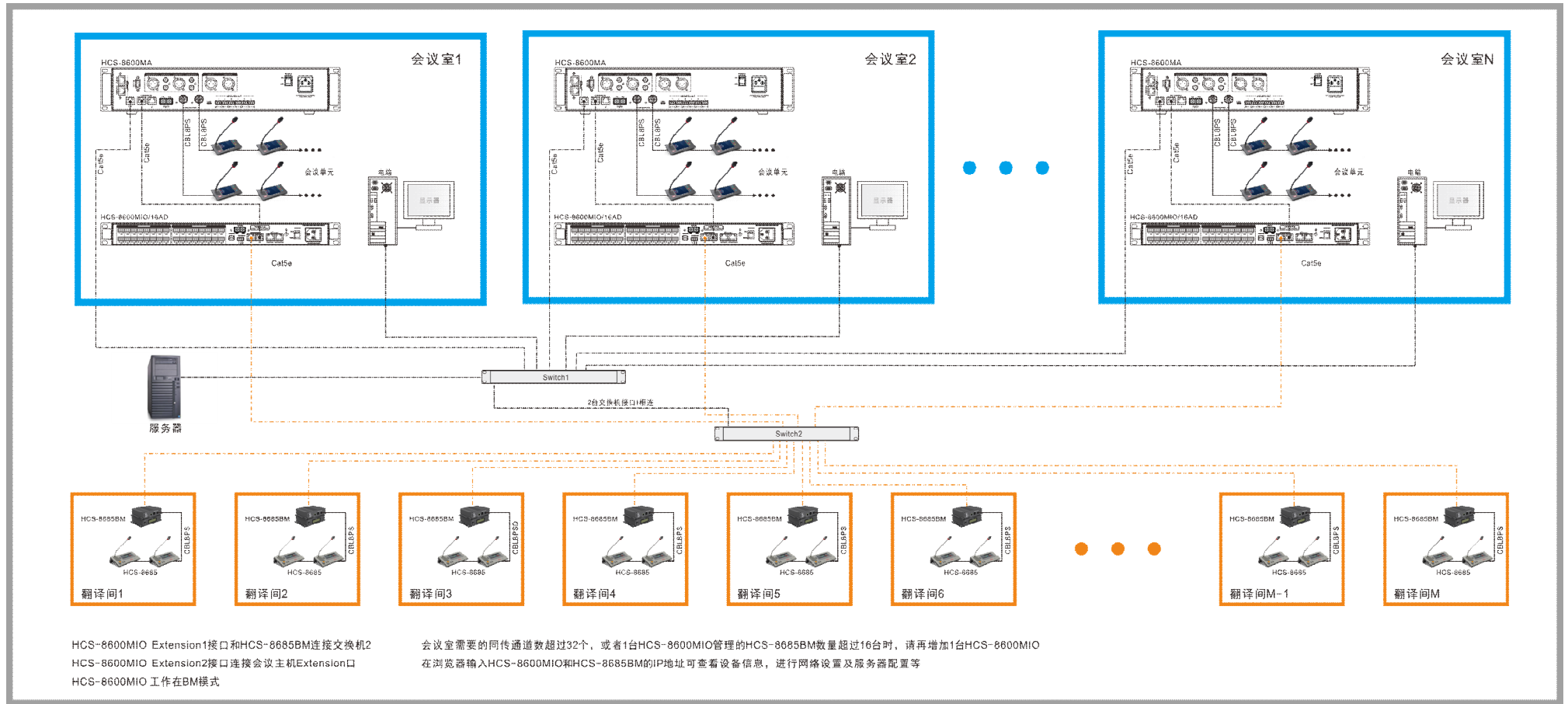
图 6.5.2-1 HCS-8685BM 译员间管理系统连接图
