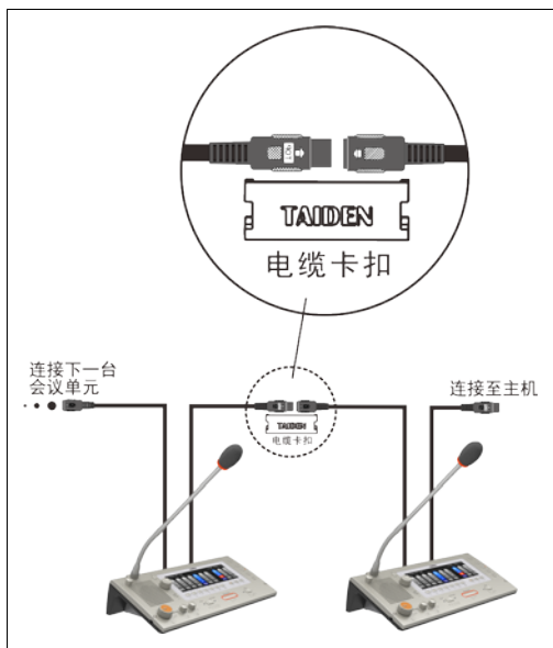
图 4.2.4 翻译单元之间“手拉手”的连接
