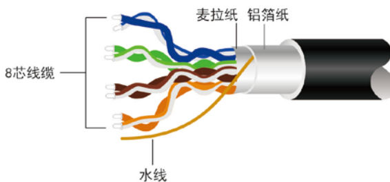
线缆如上图所示，麦拉纸和铝箔纸之间包含一条水线
