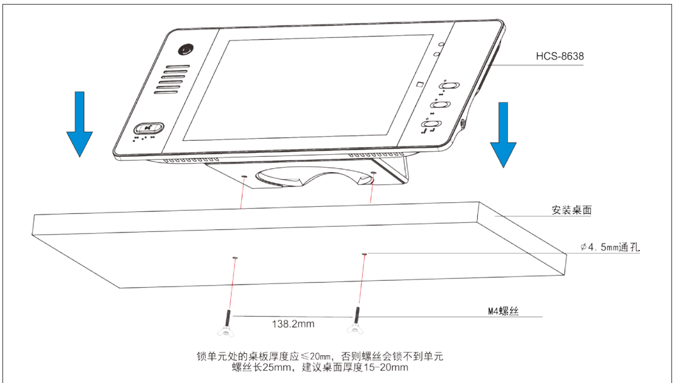
图 3.2.6 HCS-8638/50 系列无纸化多媒体终端的桌面固定安装
