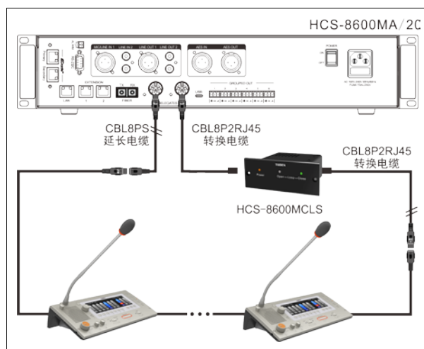
图 4.2.3 会议控制主机与 HCS-8685 翻译单元环形连接
