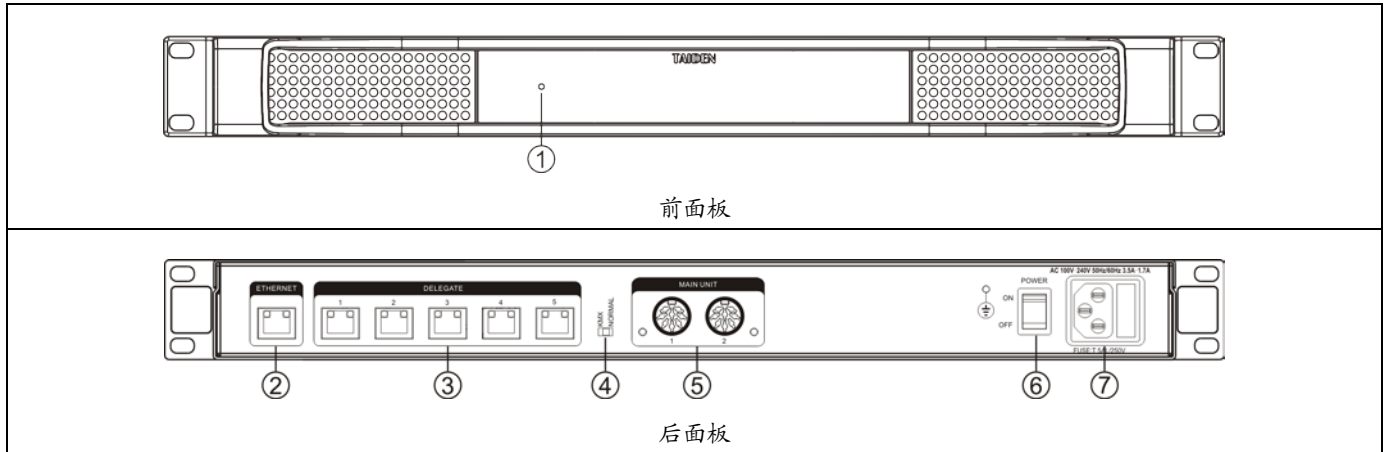
图 6.3.1 HCS-8600POE 会议专用千兆网交换机
