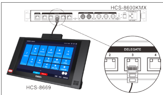
图 3.2.10 HCS-8638/8669/8668 系列无纸化多媒体会议终端与千兆网交换机的连接 (PoE 模式)
