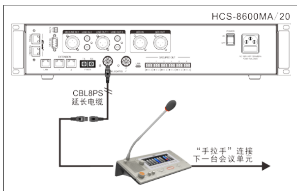
图 4.2.1 HCS-8685 翻译单元与会议控制主机或扩展主机的连接
