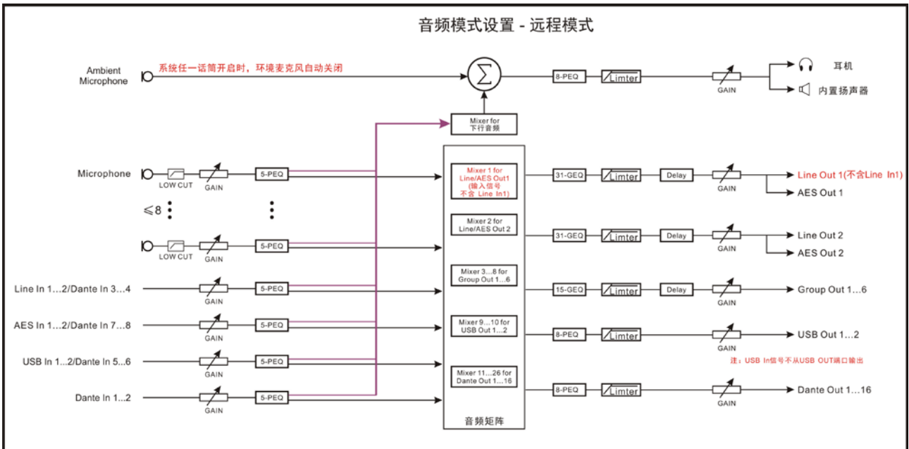
图 1.1.10 HCS-8600 系列三种音频模式信号流
