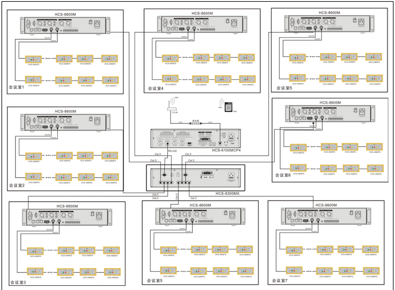
图 5.3 通过 HCS-8300MX 多会议室控制器用 Cat.5 网线将多个会议室合并/拆分
