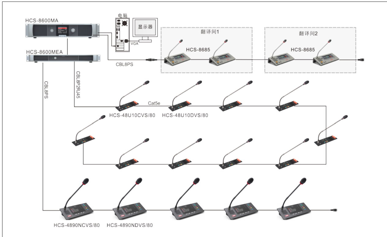
图 5.2.1 HCS-8600 系列会议系统连接实例
