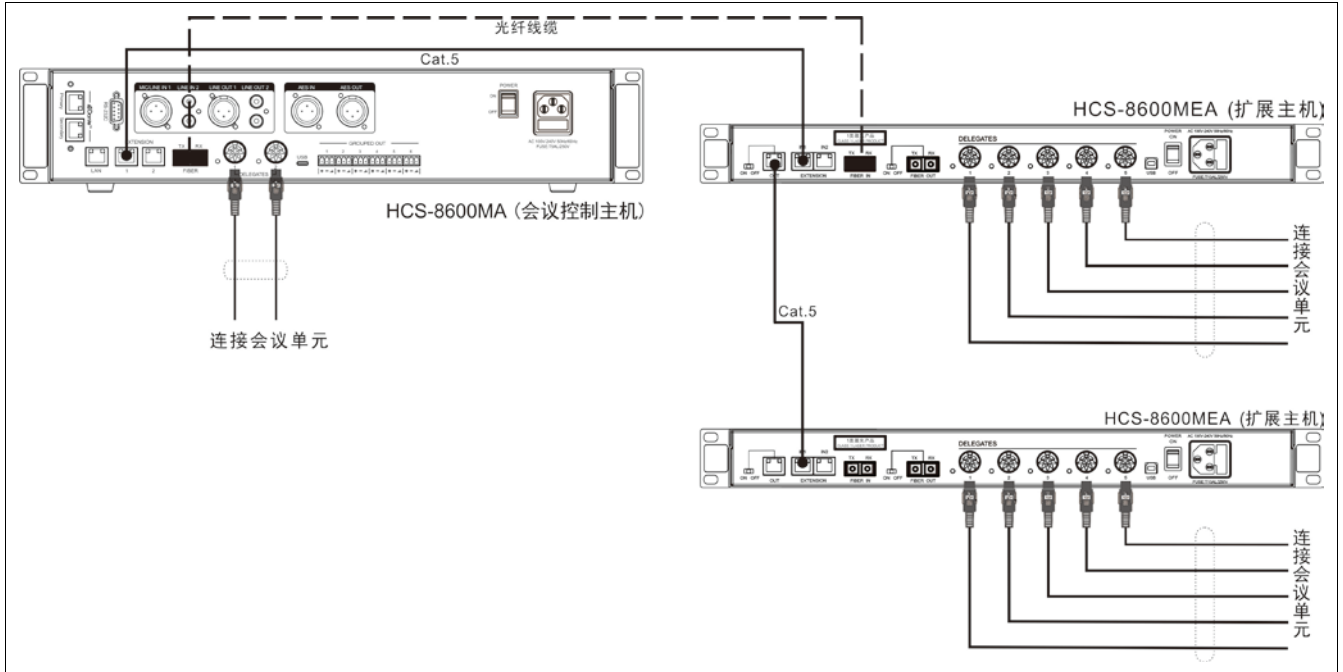
图 2.2.2 会议系统主机与扩展主机之间的连接
