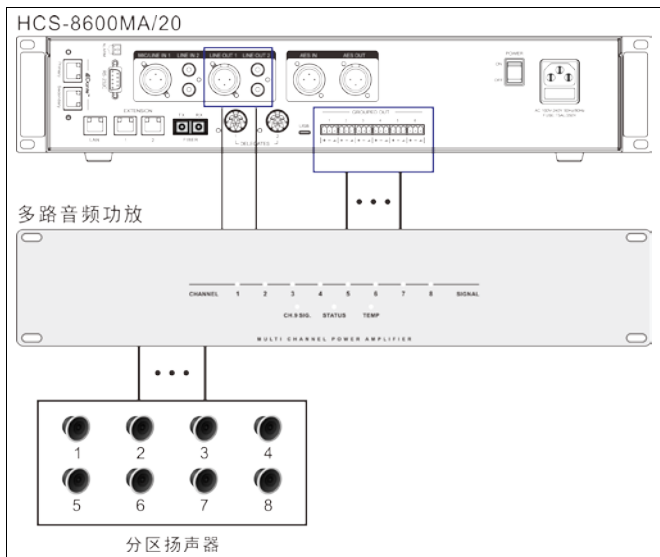
图 2.1.8 会议系统主机与功放连接
