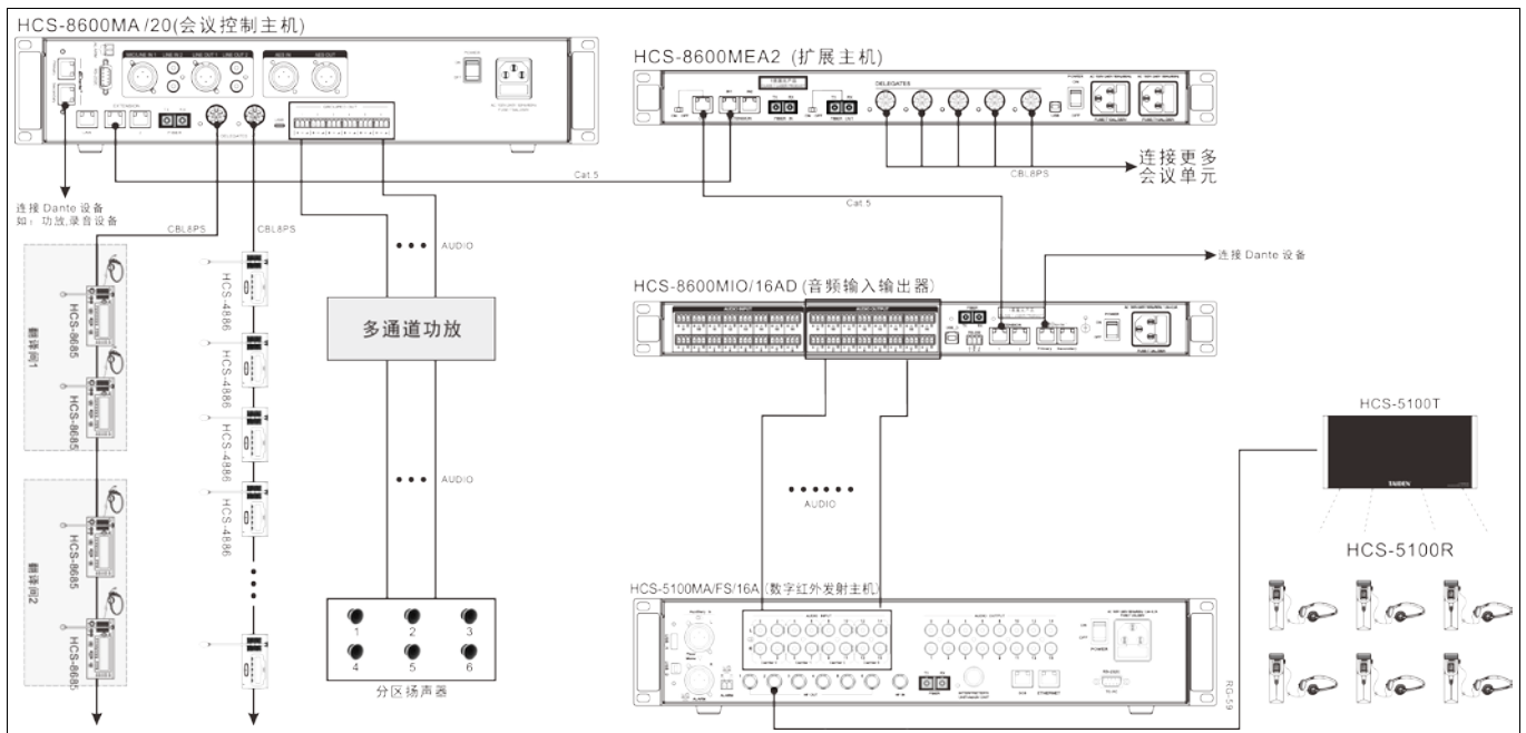
图 6.1.2 会议系统主机通过 HCS-8600MIO 连接数字红外语言分配系统
