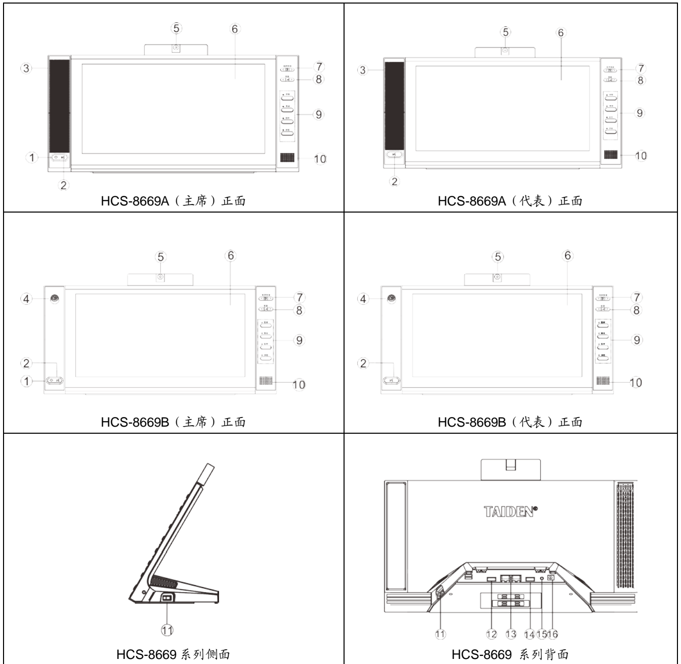
图 3.2.3 HCS-8669 系列组合式无纸化多媒体会议终端
