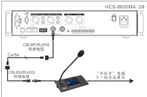
图 2.1.3 会议系统主机与会议单元（8P-DIN）的连接 2
