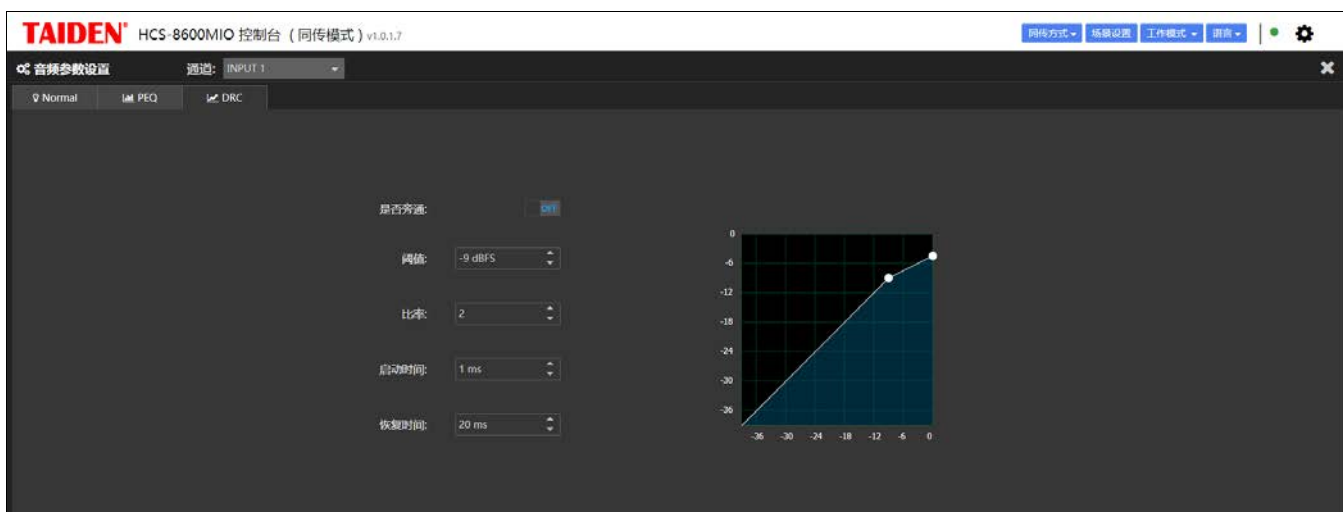
图：输入通道 DRC 设置
