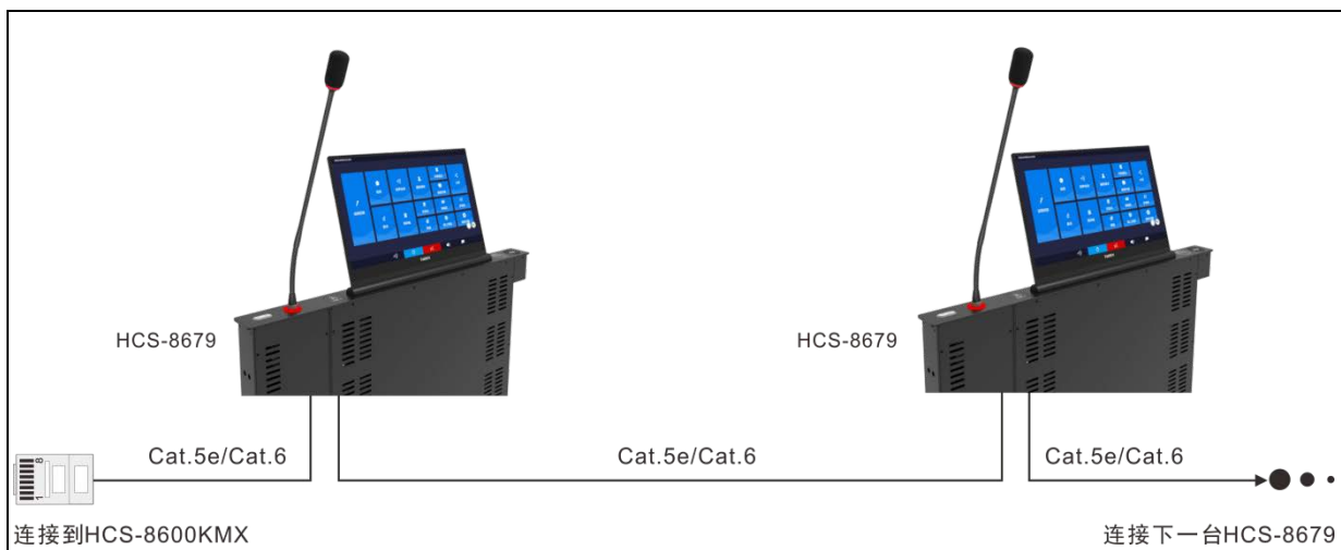
图 3.2.12 HCS-8668/8638/8669/8679 系列无纸化多媒体会议终端之间的“手拉手”连接
