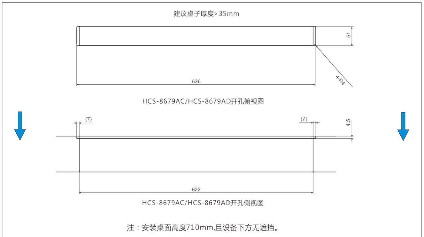
图 3.2.8 HCS-8679 系列无纸化多媒体会议终端桌面嵌入安装 (单位: mm)
