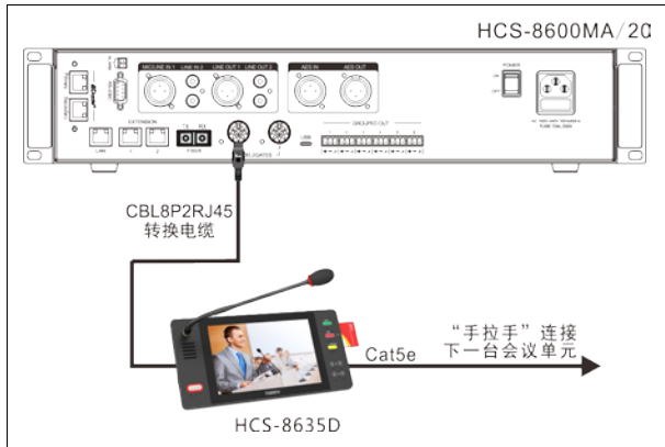
图 3.4.3 HCS-8635 系列简约型多媒体终端与会议控制主机或扩展主机的连接
