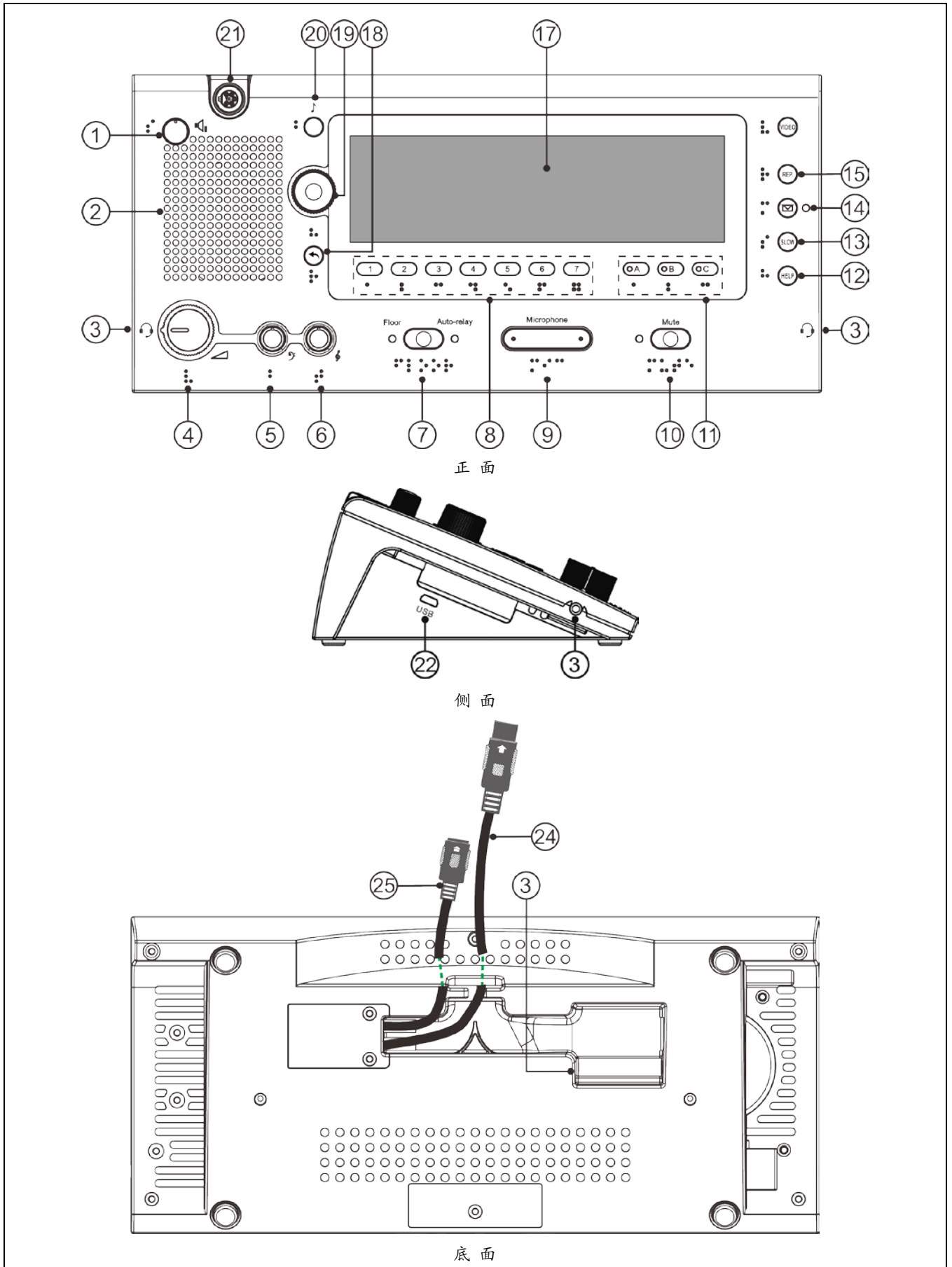
图 4.1.1 HCS-8685 翻译单元
