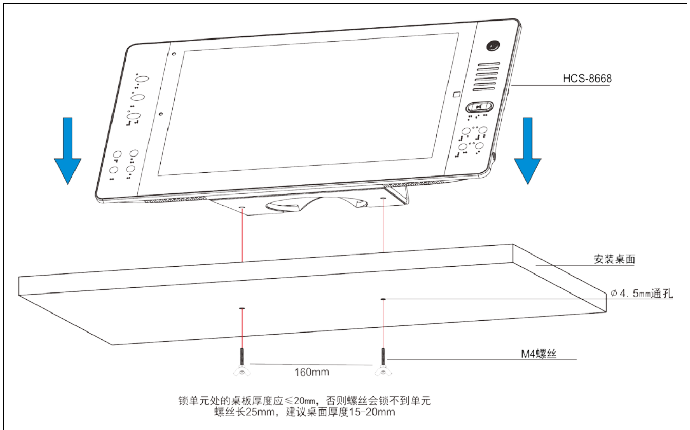
图 3.2.5 HCS-8668/50 系列无纸化多媒体终端的桌面固定安装
