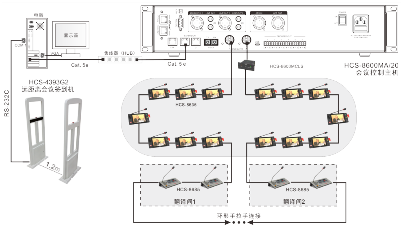
图 5.1.3 会议系统主机与会议签到系统的连接
