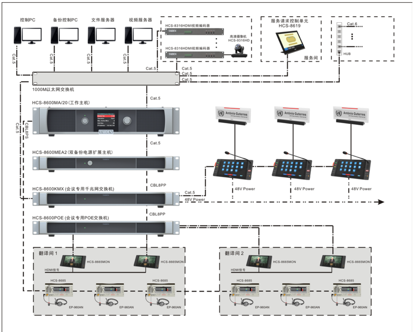
图 1.1.4 HCS-8668/50 系列无纸化多媒体会议系统连接图
