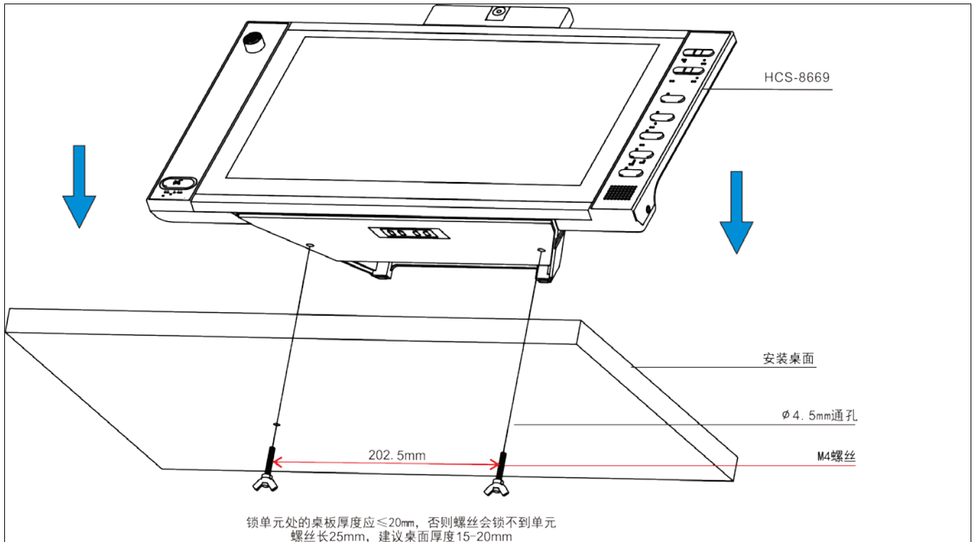
图 3.2.7 HCS-8669 系列无纸化多媒体终端的桌面固定安装
